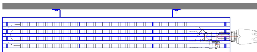
Монтажная схема настенного конвектора "Элегант 110x400-2то Терм Стен" (присоединительная резьба - 1/2")
