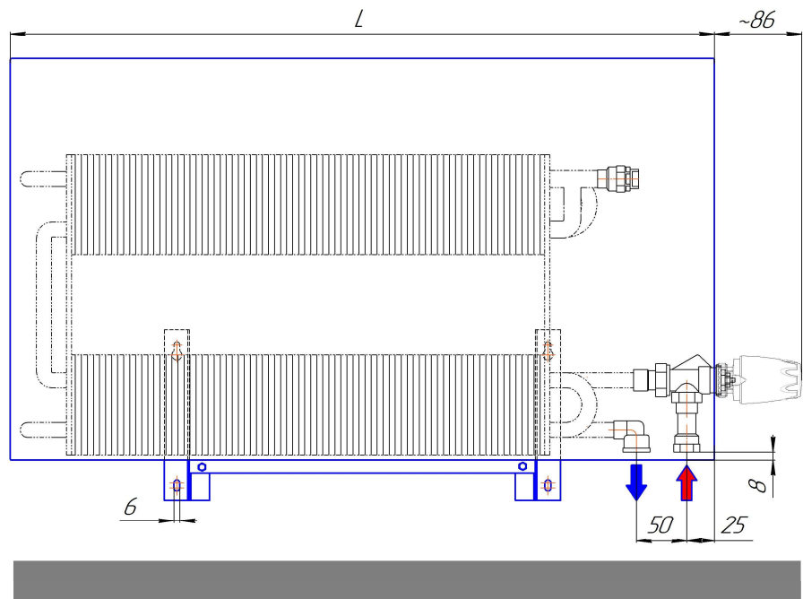
Монтажная схема настенного конвектора "Элегант 110х400-4то Терм Стен" (присоединительная резьба - 1/2")
