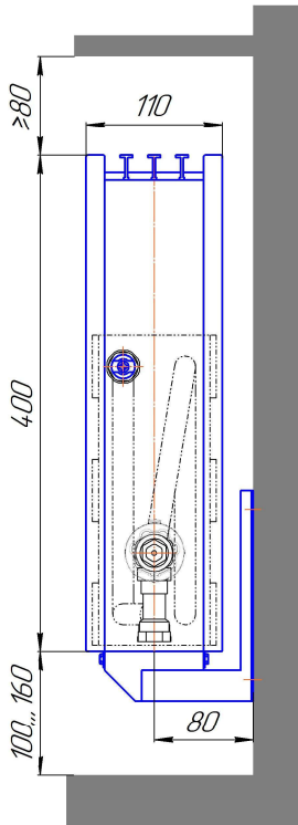
Монтажная схема настенного конвектора "Элегант 110х400-3то Терм Стен" (присоединительная резьба - 1/2")
