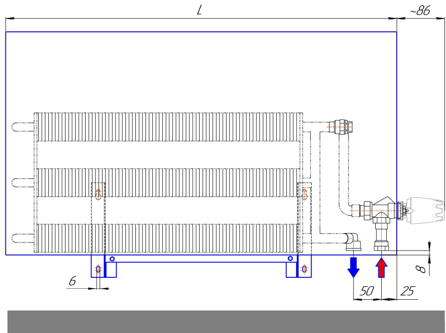
Монтажная схема настенного конвектора "Элегант 110х400-3то Терм Стен" (присоединительная резьба - 1/2")
