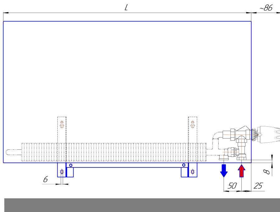
Монтажная схема настенного конвектора "Элегант 110x400-1то Терм Стен" (присоединительная резьба - 1/2")
