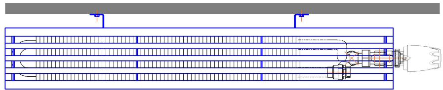
Монтажная схема настенного конвектора "Элегант 110х400-4то Терм Стен" (присоединительная резьба - 1/2")
