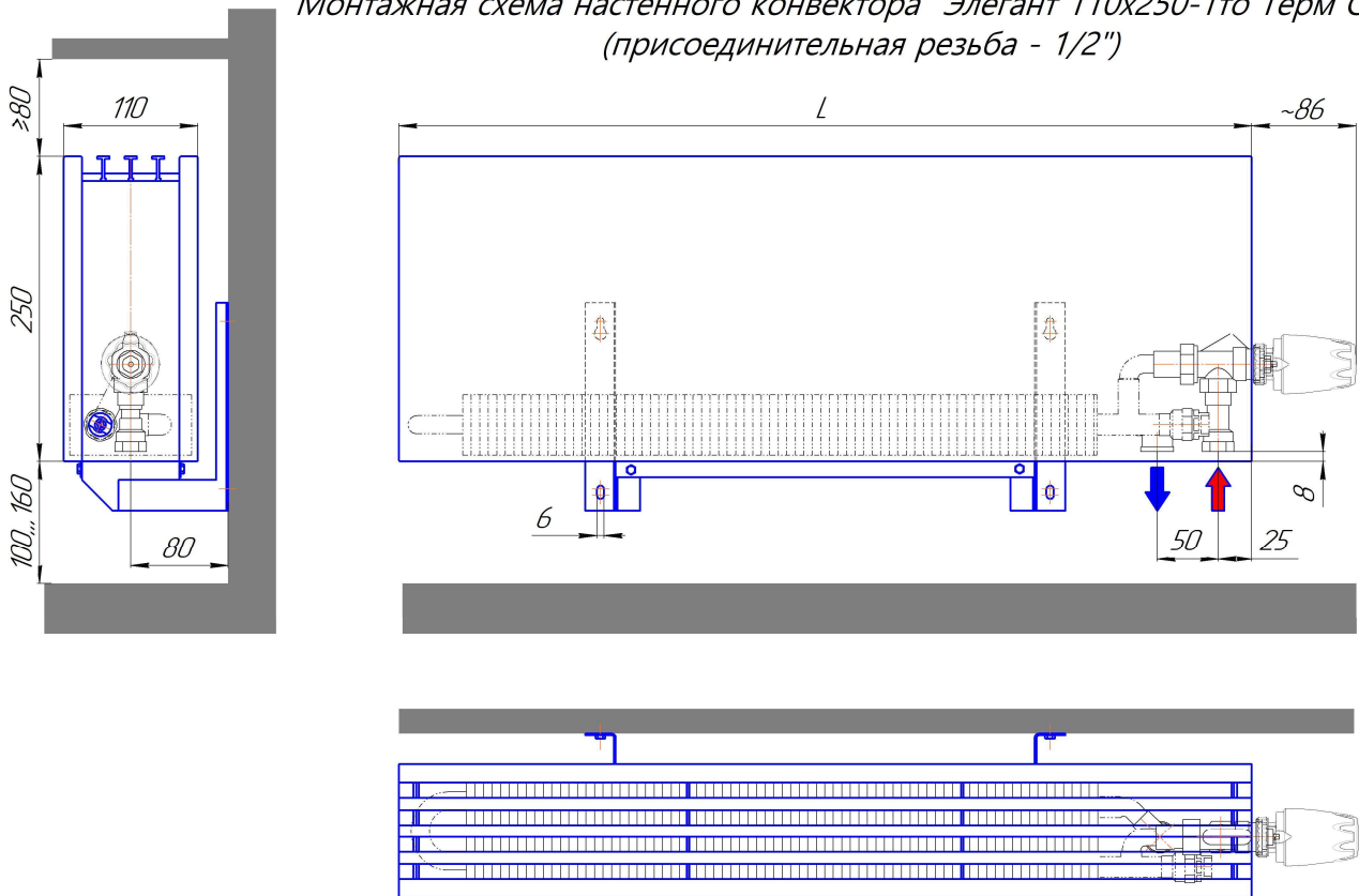
Монтажная схема настенного конвектора "Эlegant 110x250-2то Терм Стен" (присоединительная резьба - 1/2")
