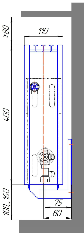
Монтажная схема настенного конвектора "Элегант 110х400-4то Терм Стен" (присоединительная резьба - 1/2")
