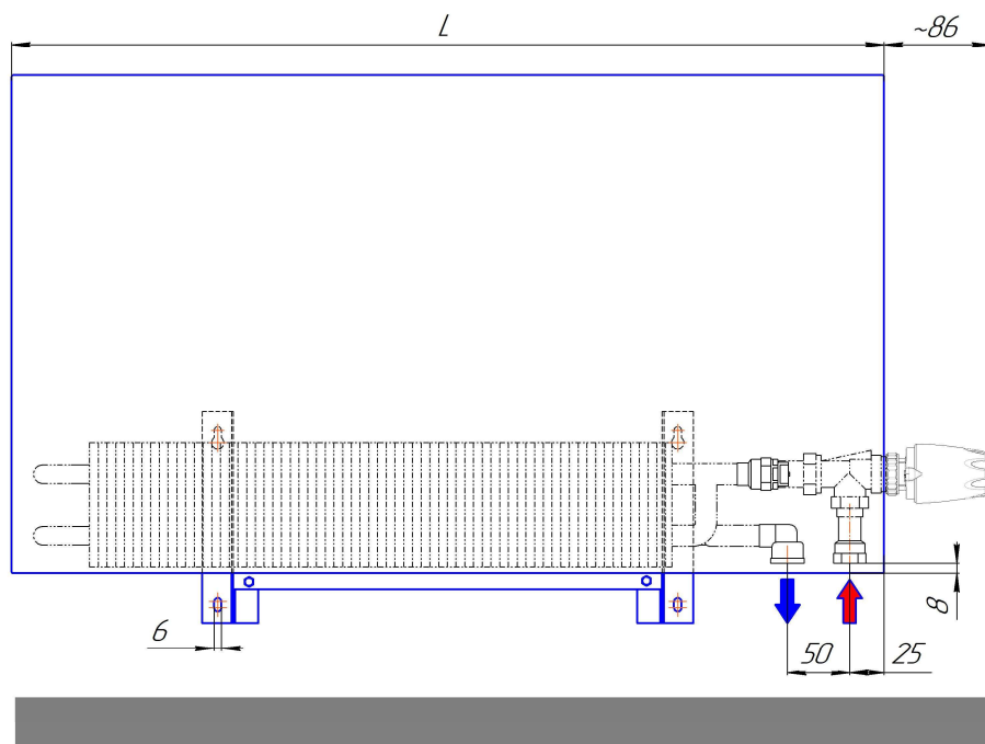
Монтажная схема настенного конвектора "Элегант 110x400-2то Терм Стен" (присоединительная резьба - 1/2")
