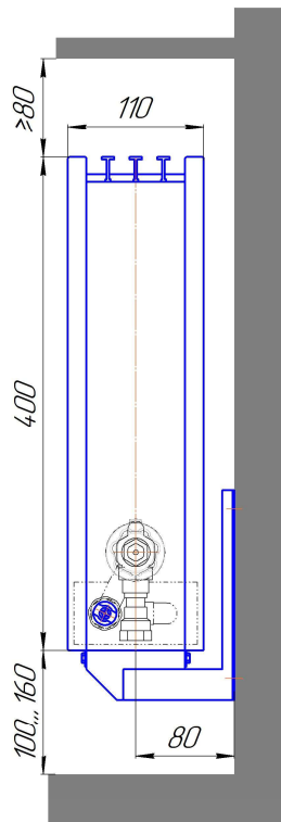
Монтажная схема настенного конвектора "Элегант 110x400-1то Терм Стен" (присоединительная резьба - 1/2")
